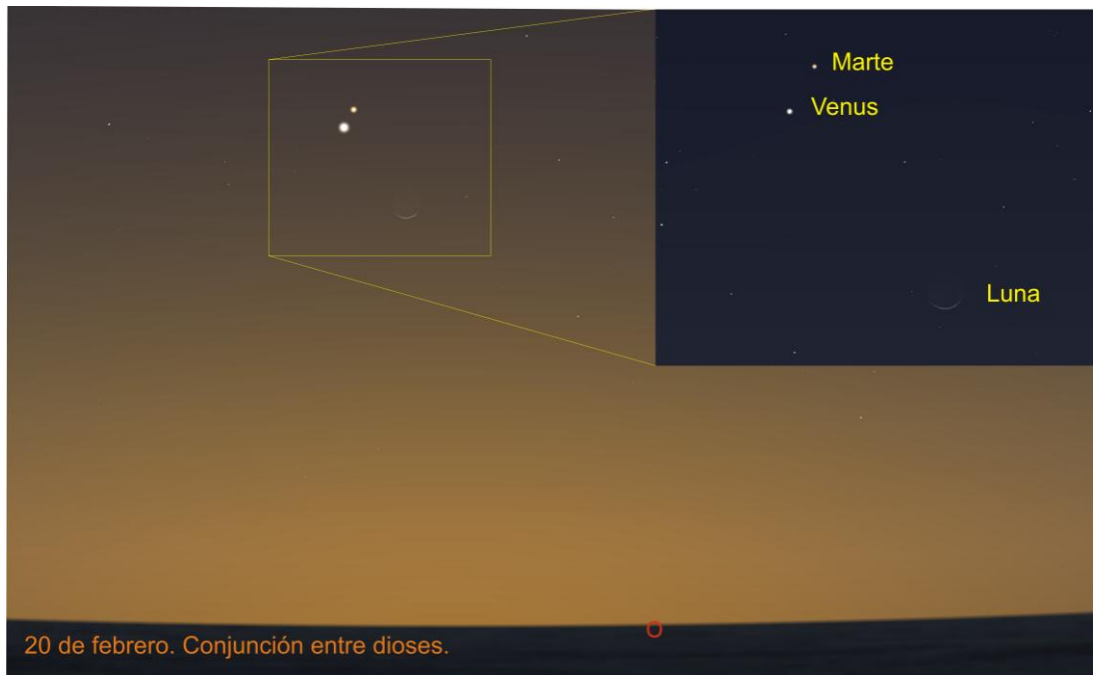
Posición de los planetas observando hacia el horizonte Oeste, tras la puesta de Sol
