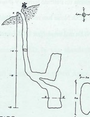
ALZADO
