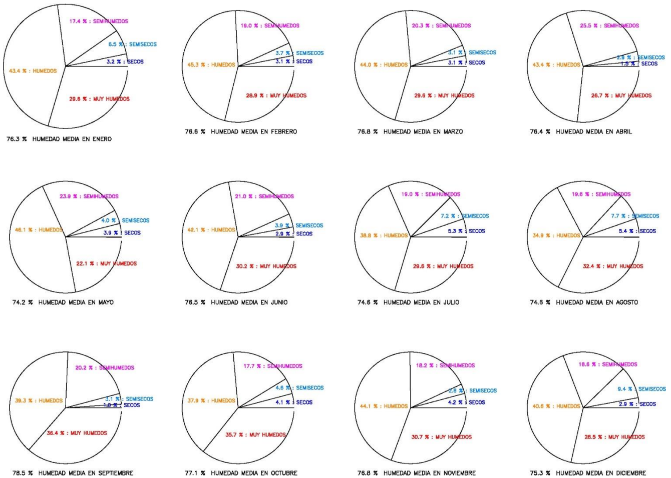
FRECUENCIAS RELATIVAS DE HUMEDADES DEL AIRE MINUTALES 2011–2021 HARÍA – LA CUESTA DEL POZO
