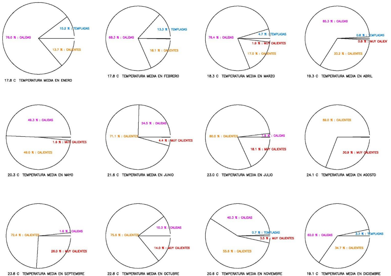
FRECUENCIAS RELATIVAS DE TEMPERATURAS DEL AIRE MINUTALES 2015–2021 YAIZA – PUERTO DE PLAYA BLANCA
