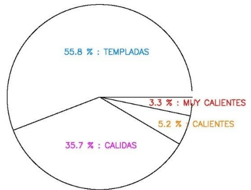
FRECUENCIAS RELATIVAS DE TEMPERATURAS DEL AIRE MINUTALES 2007–2022 HARIA – LA MONTANA
