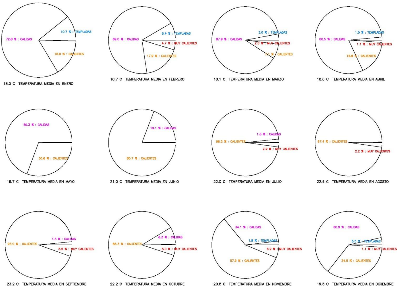
FRECUENCIAS RELATIVAS DE TEMPERATURAS DEL AIRE MINUTALES 2020–2022 TEGUISE – CALETA DE FAMARA
