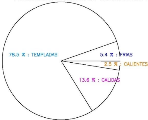
FRECUENCIAS RELATIVAS DE TEMPERATURAS DEL AIRE MINUTALES 2007–2022 HARIA – LA MONTANA
