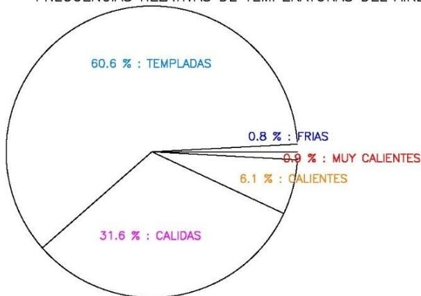
FRECUENCIAS RELATIVAS DE TEMPERATURAS DEL AIRE MINUTALES 2015–2021 TÍAS – LAS VEGAS
