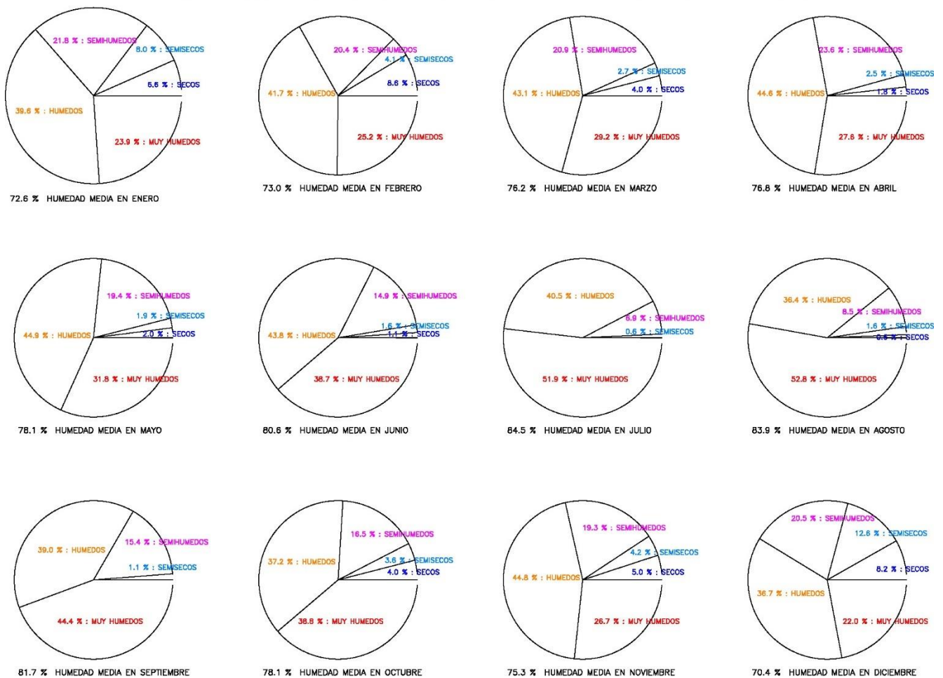
FRECUENCIAS RELATIVAS DE HUMEDADES DEL AIRE MINUTALES 2011–2021 TINAJO – VIRGEN DE LOS DOLORES
