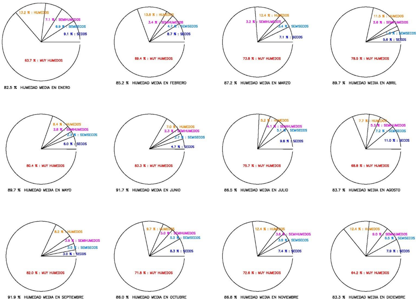
FRECUENCIAS RELATIVAS DE HUMEDADES DEL AIRE MINUTALES 2007–2022 HARÍA – LA MONTAÑA
