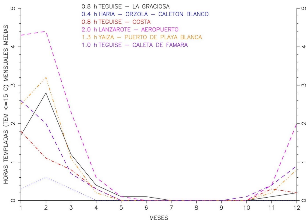
Perfiles de las horas frías y templadas mensuales medias en la franja costera lanzaroteña
