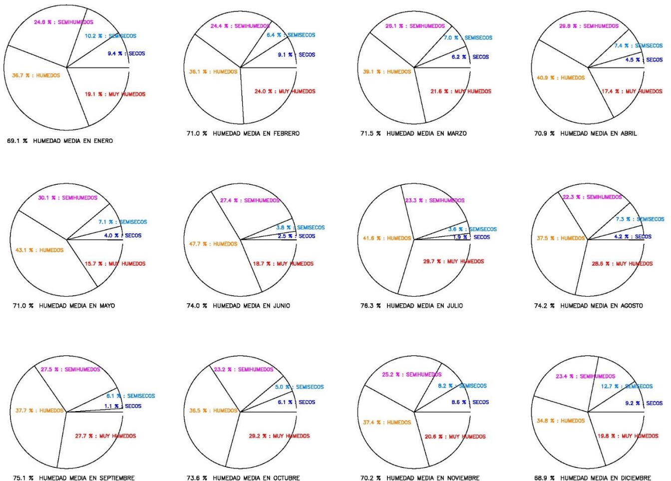
FRECUENCIAS RELATIVAS DE HUMEDADES DEL AIRE MINUTALES 2007-2020 LA GERIA
