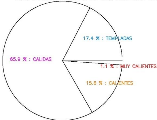
FRECUENCIAS RELATIVAS DE TEMPERATURAS DEL AIRE MINUTALES 2007-2022 ARRECIFE – LA GRANJA
