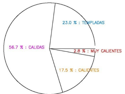
FRECUENCIAS RELATIVAS DE TEMPERATURAS DEL AIRE MINUTALES 2015–2021 TÍAS – LAS VEGAS
