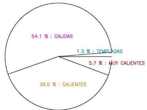
FRECUENCIAS RELATIVAS DE TEMPERATURAS DEL AIRE MINUTALES 2007-2022 ARRECIFE – LA GRANJA
