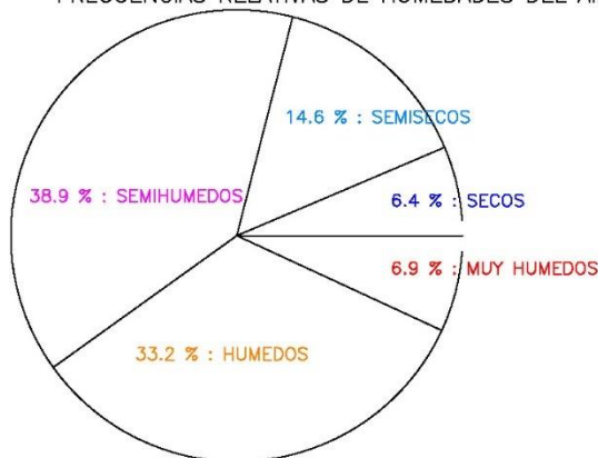
FRECUENCIAS RELATIVAS DE HUMEDADES DEL AIRE MINUTALES
