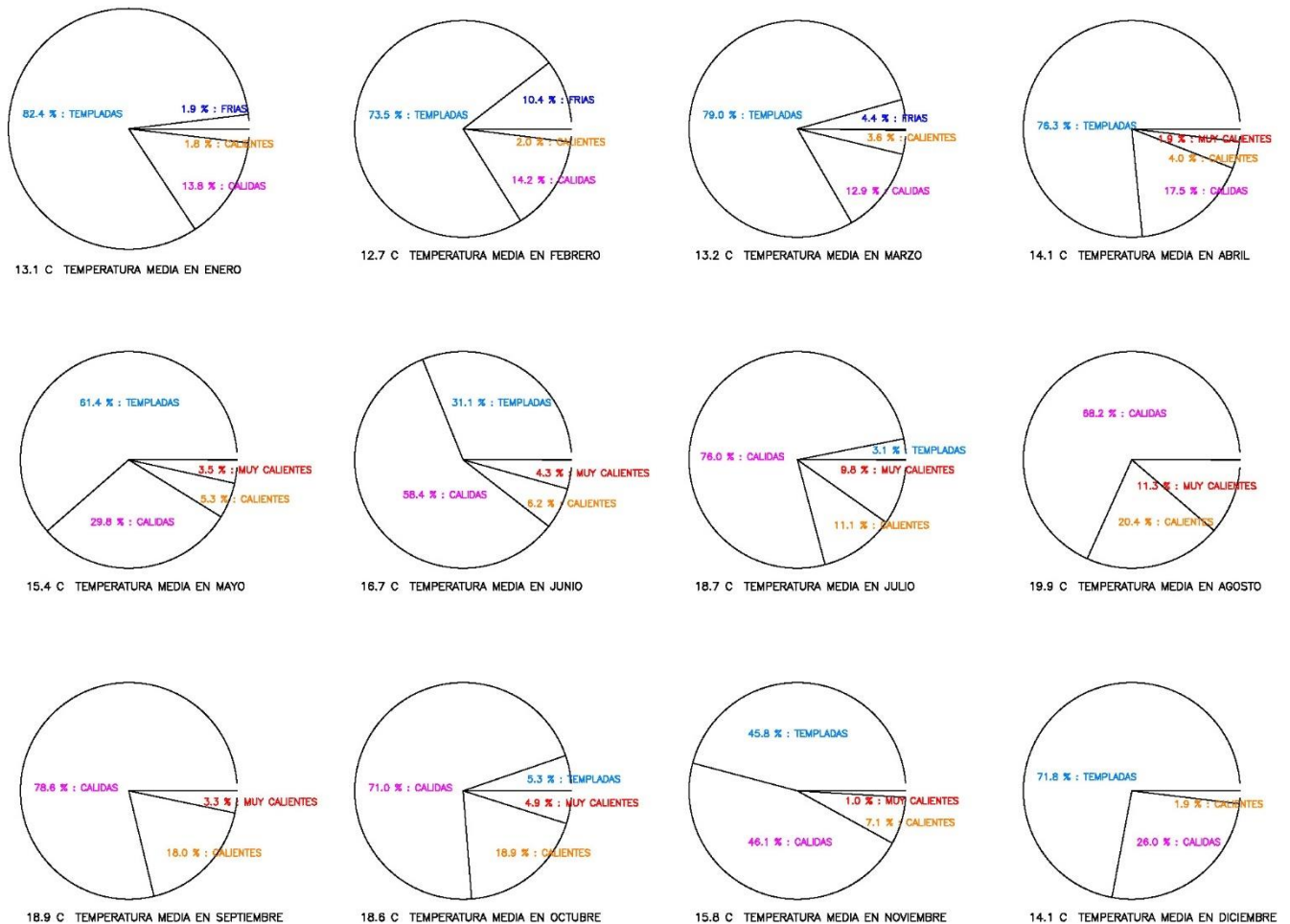
FRECUENCIAS RELATIVAS DE TEMPERATURAS DEL AIRE MINUTALES 2007–2022 HARIA – LA MONTANA
