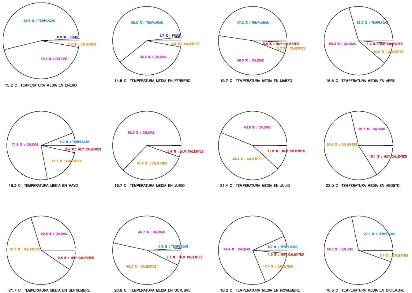
FRECUENCIAS RELATIVAS DE TEMPERATURAS DEL AIRE MINUTALES 2011–2021 HARIA – LA CUESTA DEL POZO
