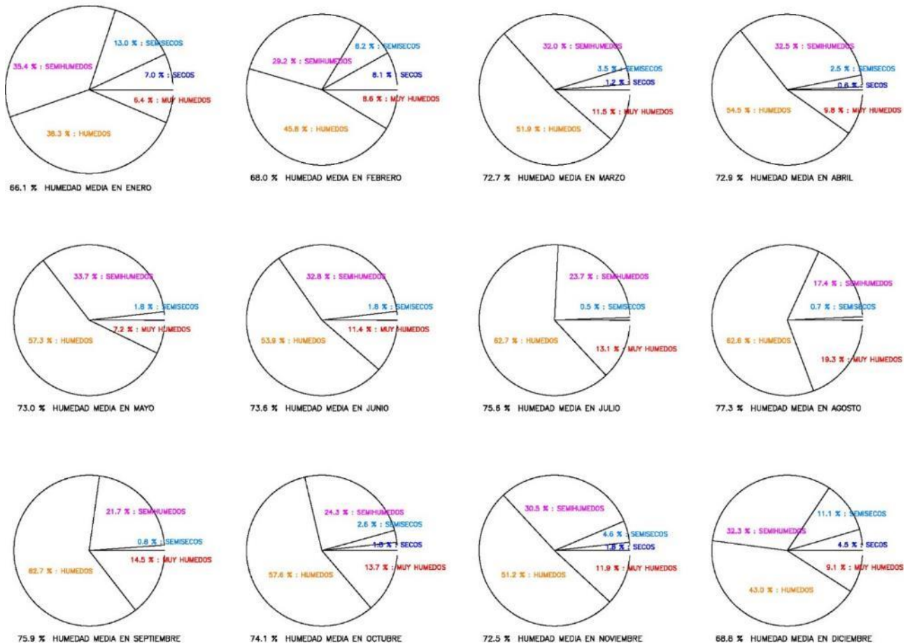
FRECUENCIAS RELATIVAS DE HUMEDADES DEL AIRE MINUTALES
