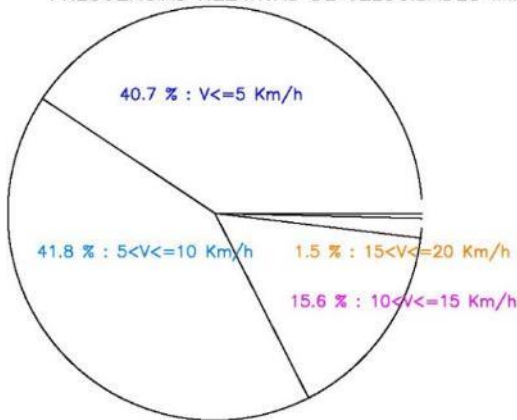
FRECUENCIAS RELATIVAS DE VELOCIDADES MINUTALES DEL VIENTO 2014–2022 LOS SILOS
