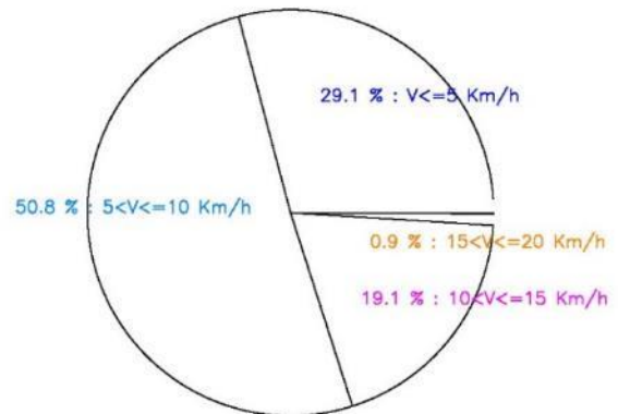
FRECUENCIAS RELATIVAS DE VELOCIDADES MINUTALES DEL VIENTO 2014–2022 LOS SILOS
