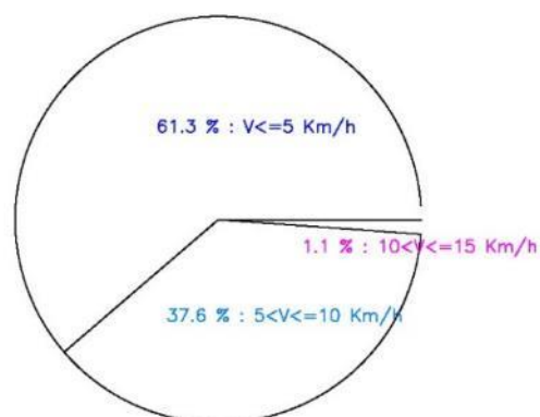
4.4 Km/h VELOCIDAD DEL VIENTO EN PRIMAVERA
