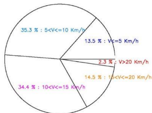
FRECUENCIAS RELATIVAS DE VELOCIDADES MINUTALES DEL VIENTO 2001–2022 BUENAVISTA DEL NORTE
