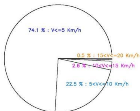
3.9 Km/h VELOCIDAD DEL VIENTO EN OTONO
