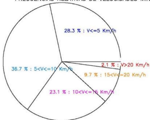
FRECUENCIAS RELATIVAS DE VELOCIDADES MINUTALES DEL VIENTO 2001–2022 BUENAVISTA DEL NORTE
