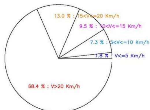
FRECUENCIAS RELATIVAS DE VELOCIDADES MINUTALES DEL VIENTO 2021-2023 BUENAVISTA NORTE - PUNTA TENO
