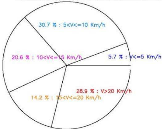
FRECUENCIAS RELATIVAS DE VELOCIDADES MINUTALES DEL VIENTO 2011-2019 LOS SILOS – DEPURADORA
