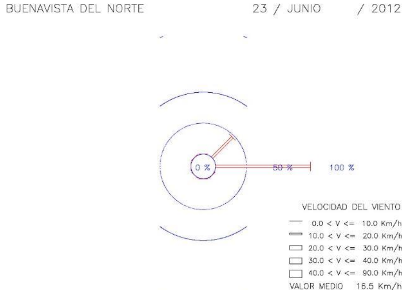
Rosa de viento en la costa de Buenavista del Norte el 23 de junio de 2012
