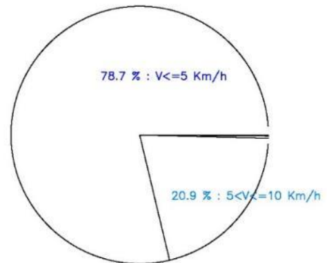
FRECUENCIAS RELATIVAS DE VELOCIDADES MINUTALES DEL VIENTO 2004–2022 ICOD DE LOS VINOS – REDONDO
