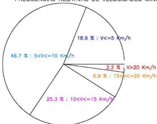
FRECUENCIAS RELATIVAS DE VELOCIDADES MINUTALES DEL VIENTO 2005-2022 LOS REALEJOS - ICOD EL ALTO
