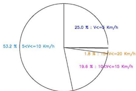
FRECUENCIAS RELATIVAS DE VELOCIDADES MINUTALES DEL VIENTO 2019–2023 GARACHICO – LA MONTANETA
