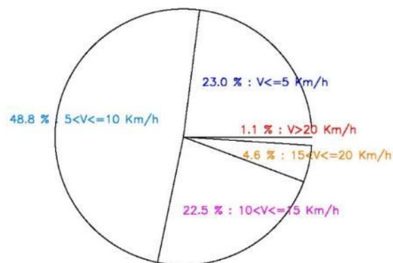
FRECUENCIAS RELATIVAS DE VELOCIDADES MINUTALES DEL VIENTO 2005-2022 LOS REALEJOS - ICOD EL ALTO
