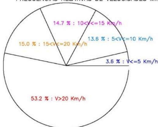
FRECUENCIAS RELATIVAS DE VELOCIDADES MINUTALES DEL VIENTO 2021-2023 BUENAVISTA NORTE - PUNTA TENO
