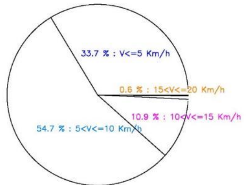
FRECUENCIAS RELATIVAS DE VELOCIDADES MINUTALES DEL VIENTO 2016–2022 EL TANQUE – RUIGOMEZ
