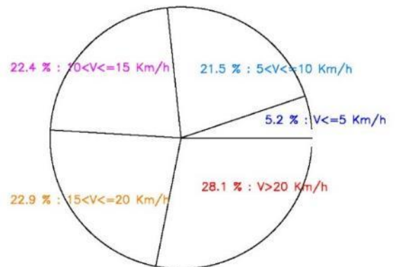
FRECUENCIAS RELATIVAS DE VELOCIDADES MINUTALES DEL VIENTO 2011-2019 LOS SILOS – DEPURADORA
