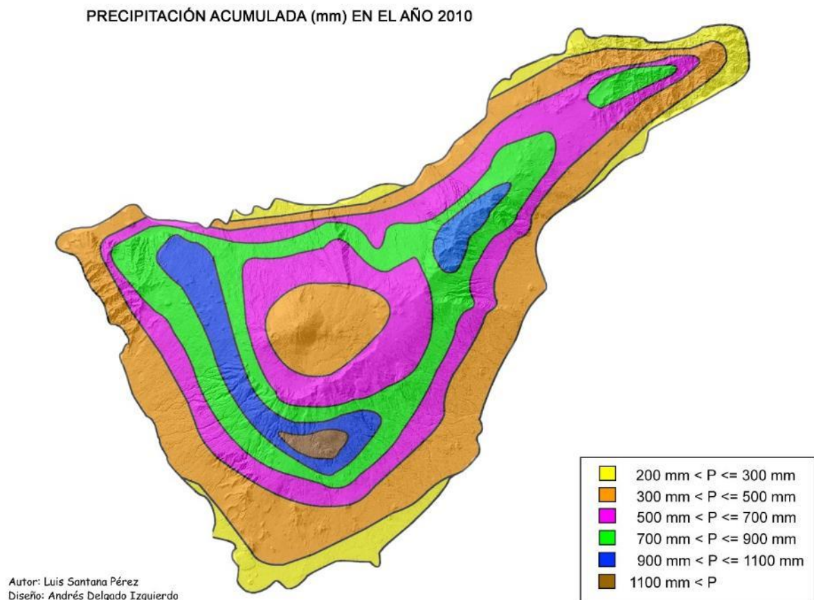
Mapa esquemático de isoyetas 2010, el año más lluvioso
