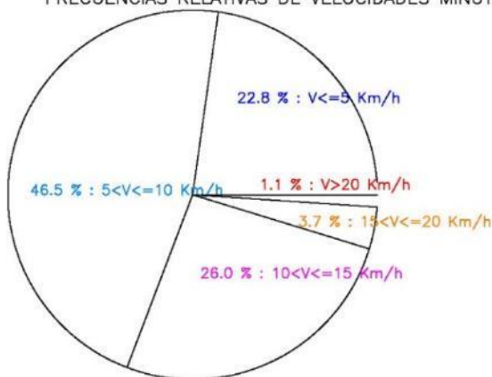
FRECUENCIAS RELATIVAS DE VELOCIDADES MINUTALES DEL VIENTO 2019–2023 GARACHICO – LA MONTANETA
