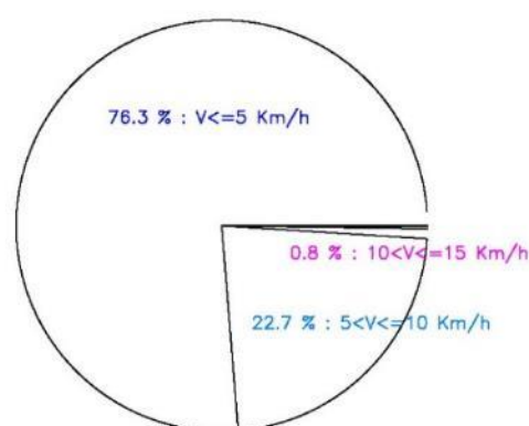
4.0 Km/h VELOCIDAD DEL VIENTO EN OTONO
