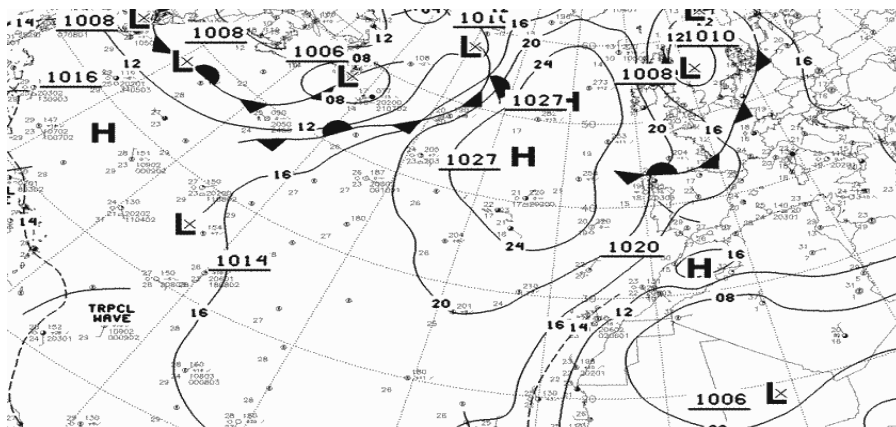
Situación barométrica de día muy caluroso y seco el 12 de agosto de 2010. Presencia de aire sahariano
