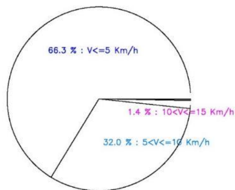
4.4 Km/h VELOCIDAD DEL VIENTO EN PRIMAVERA
