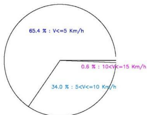
4.3 Km/h VELOCIDAD DEL VIENTO EN OTONO
