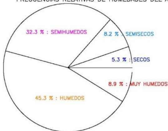
FRECUENCIAS RELATIVAS DE HUMEDADES DEL AIRE MINUTALES
