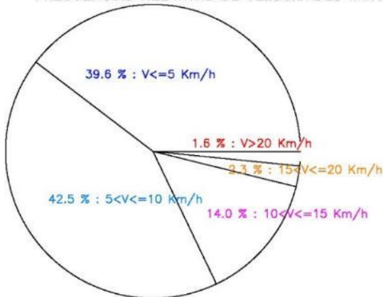
FRECUENCIAS RELATIVAS DE VELOCIDADES MINUTALES DEL VIENTO 2016–2022 EL TANQUE – RUIGOMEZ
