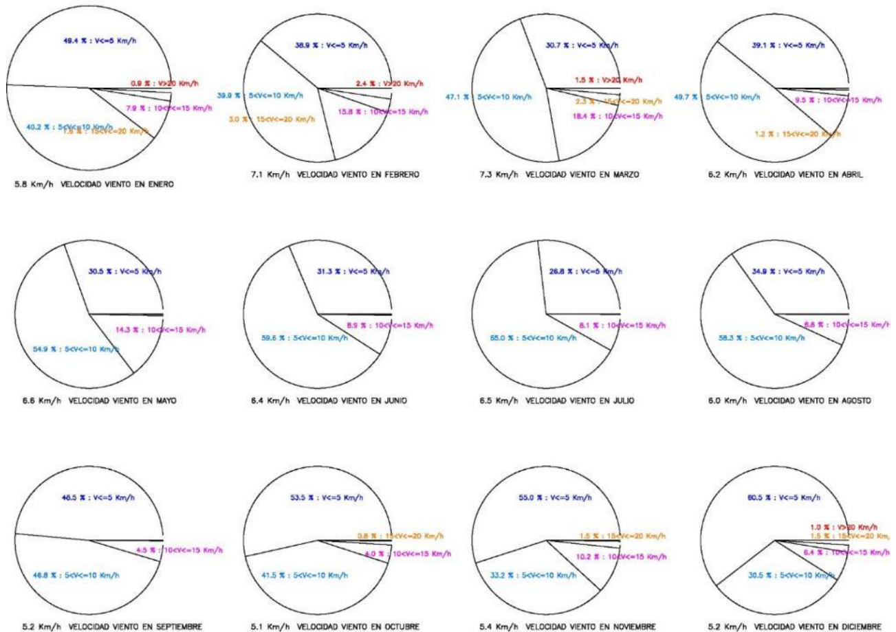
FRECUENCIAS RELATIVAS DE VELOCIDADES MINUTALES DEL VIENTO 2016–2022 EL TANQUE – RUIGÓMEZ
