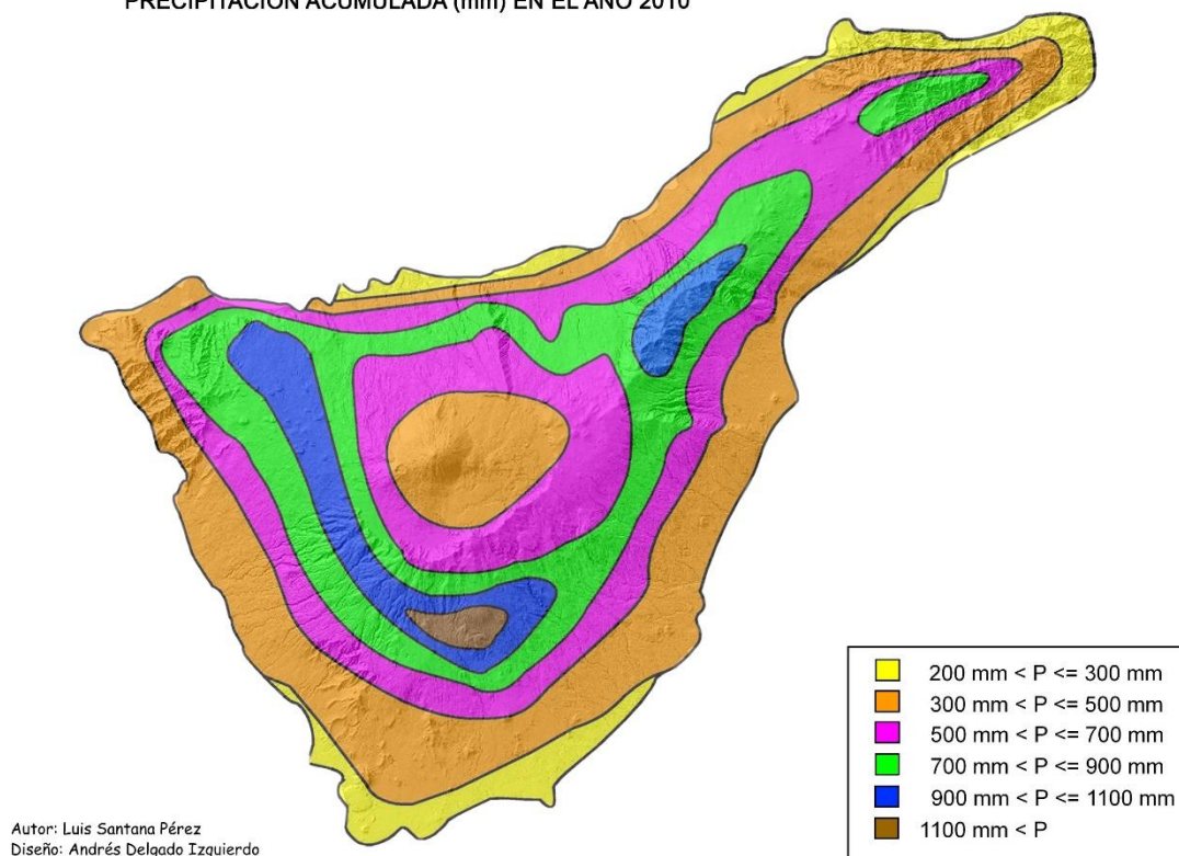
PRECIPITACIÓN ACUMULADA (mm) EN EL AÑO 2010
