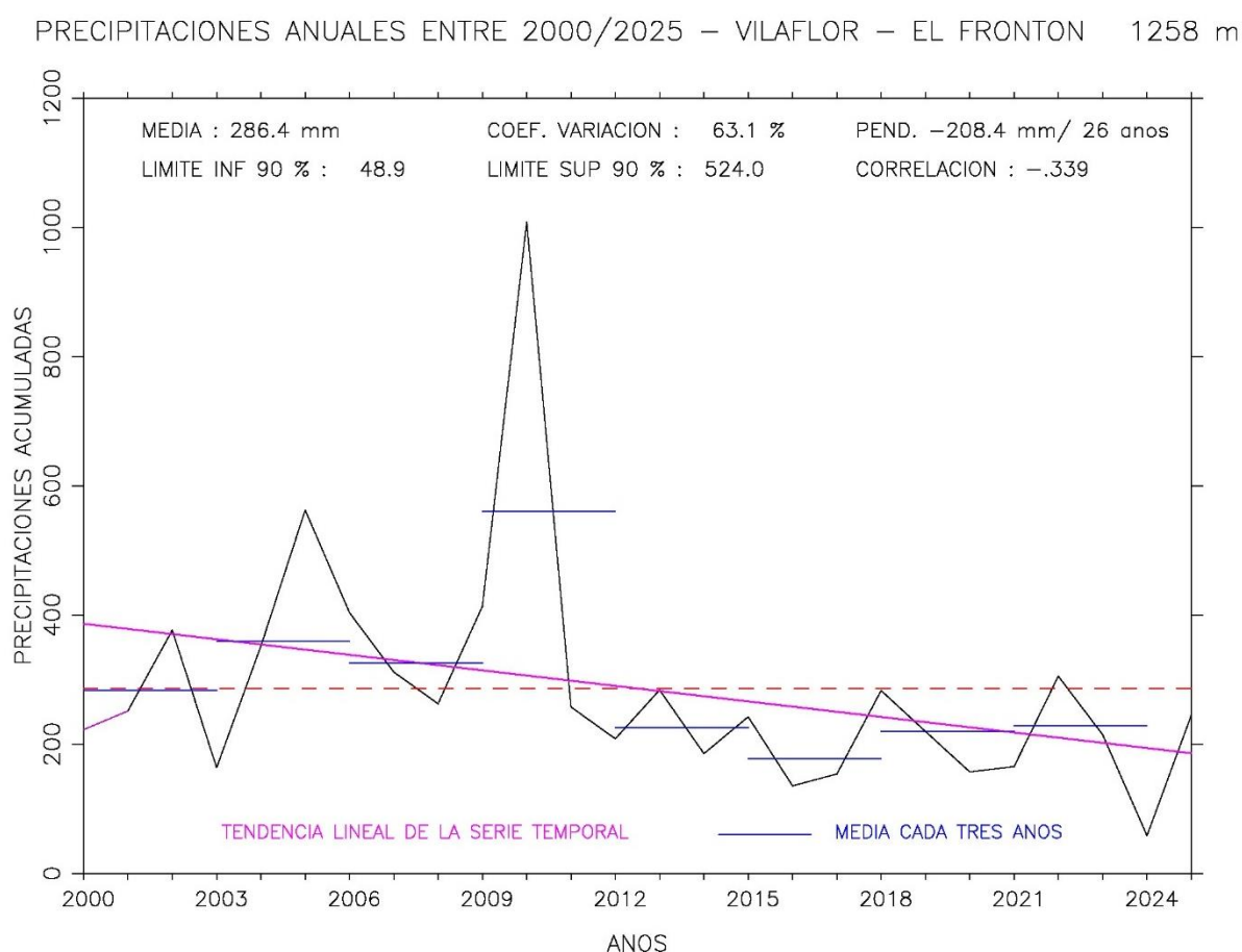
Tendencia de las precipitaciones anuales acumuladas
